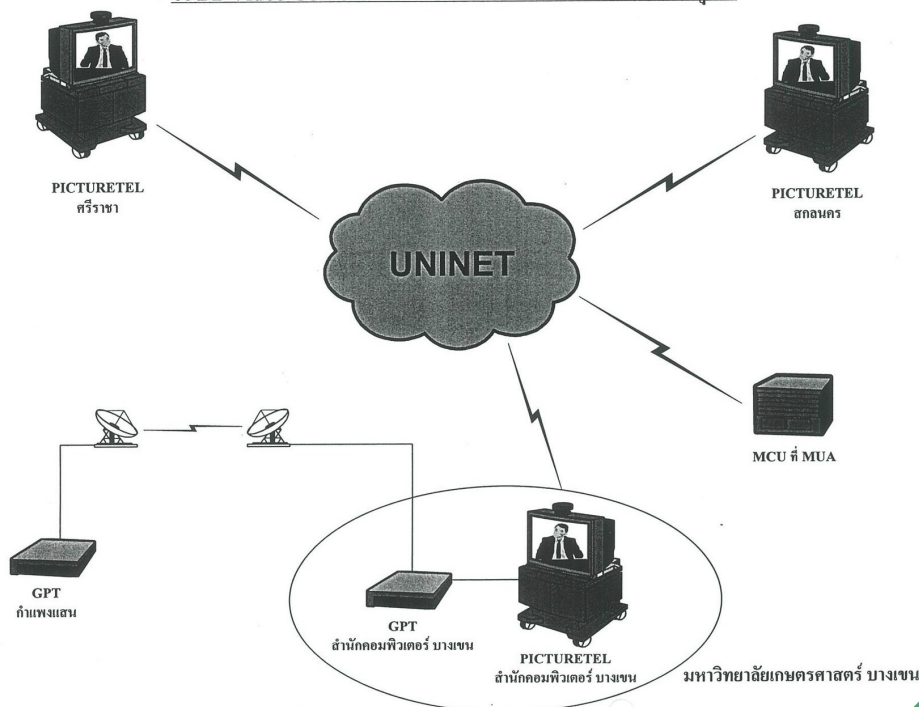
ระบบ Video Conference ที่มหาวิทยาลัยเกษตรศาสตร์ ปัจจุบัน
