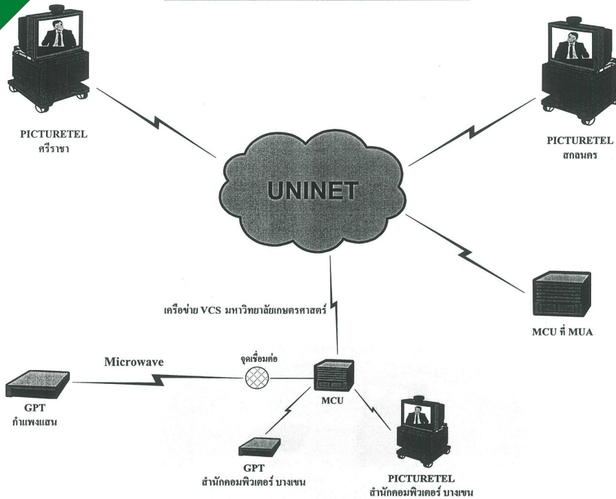
ระบบการต่อ Video Conference ในงานวันเปิด
